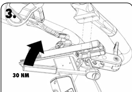
LLAVE HEXAGONAL ESFÉRICA DE 6 MM
